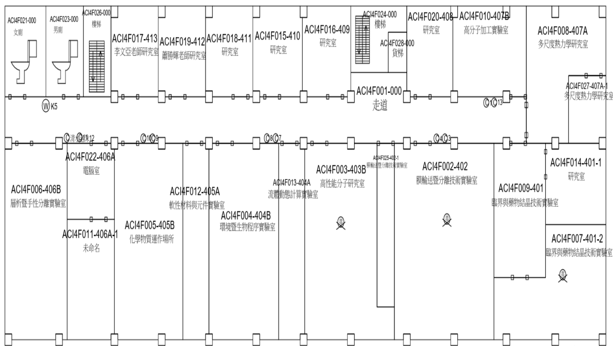
化工館 4F平面圖
