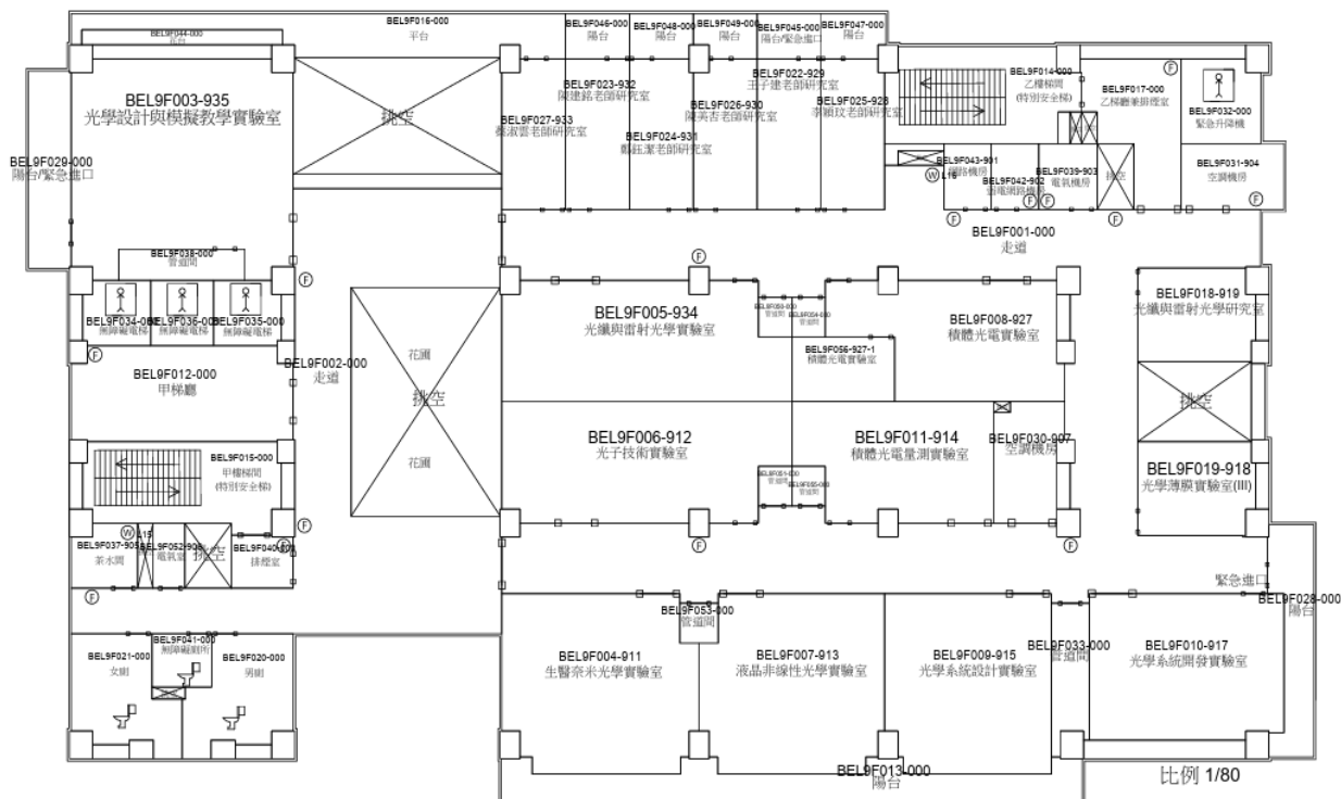
億光大樓 9F平面圖
